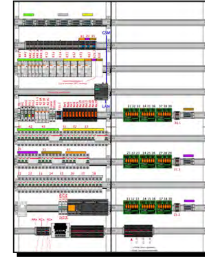
6305 -ryhmäkeskus -K/P-kontaktorit -Logo8 kotiautomaatio - 27-kanavainen valo-ohjaus -asennustilaa
