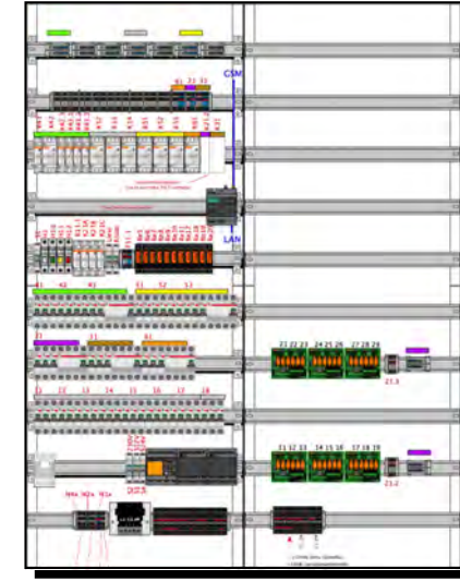
6304 -ryhmäkeskus -K/P-kontaktorit -Logo8 kotiautomaatio - 18-kanavainen valo-ohjaus -asennustilaa
