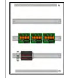
6299 -uppoasennus - 9-kanavainen valo-ohjaus
