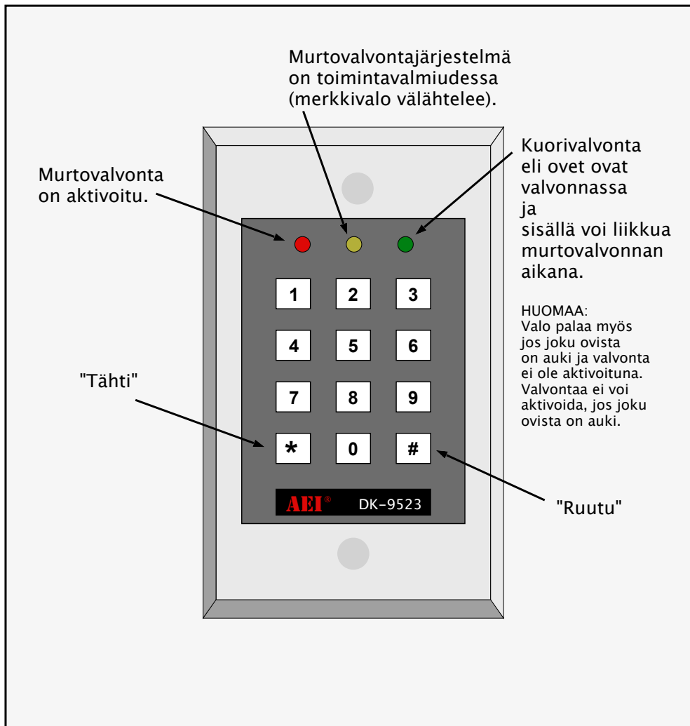
KUVA 7: Talon murtohälytysjärjestelmän käyttölaite
